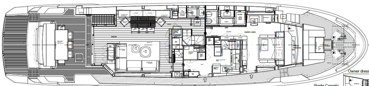
Ponte Coperta Main deck
